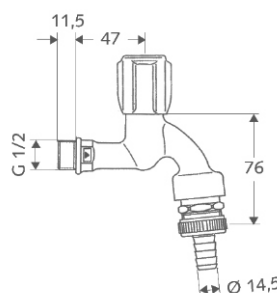
Výtokový ventil COMFORT s rukojetí COMFORT a vrškem s tukovou komorou.
