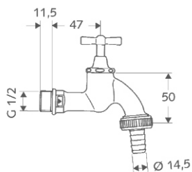
Výtokový ventil vršek s otočnou páčkou
